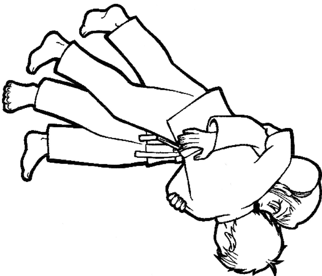
Uki-Goshi
